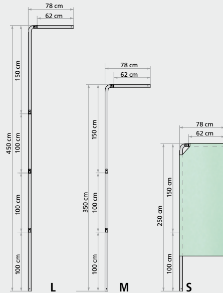
Fahnenstange Economy mit Ausleger
